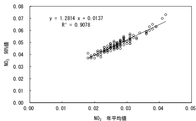
図2.1-7(1) 二酸化窒素の日平均値の年間98%値への変換式相関図(自動車排出ガス測定局) (N=130)
