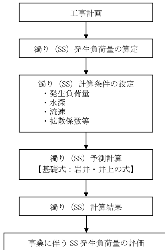
図 9.2-9 工事の施行中における濁り（SS）の予測手順
