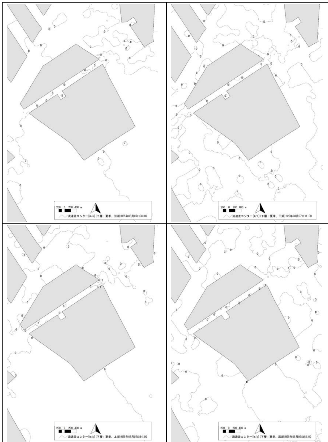
図 9.2-14 (2)潮流の変化 (将来予測値-現況再現値) (下層：夏季、平成 25 年 8 月 7 日) (左上：引潮時 右上：干潮時 左下：上潮時 右下：満潮時)
